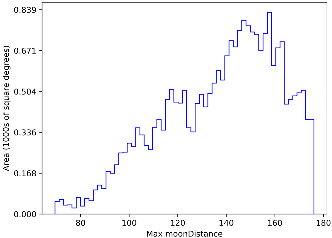
noroll_mjdp365_v3.4_10yrs All sky y band: Max moonDistance
