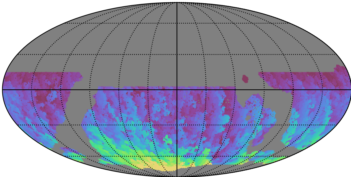
noroll_mjdp365_v3.4_10yrs WFD y band: Max HA
