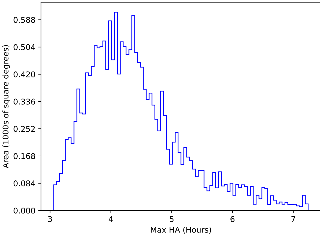
noroll_mjdp365_v3.4_10yrs WFD y band: Max HA
