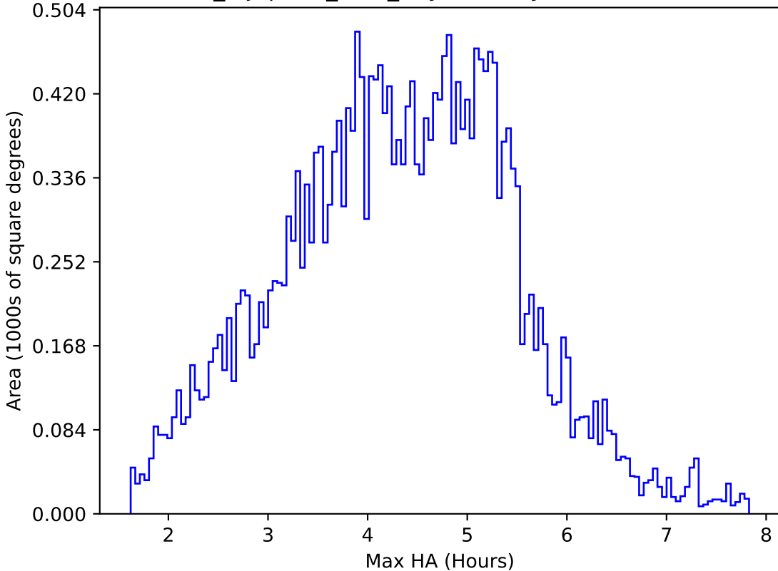
noroll_mjdp365_v3.4_10yrs All sky z band: Max HA
