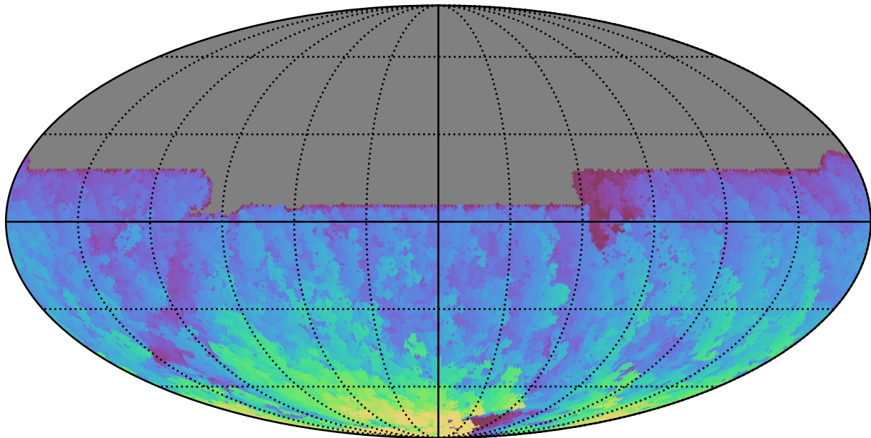
noroll_mjdp365_v3.4_10yrs All sky y band: Max HA
