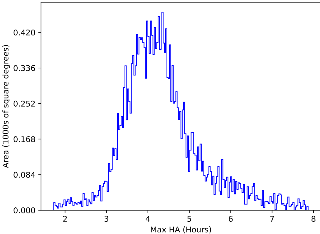
noroll_mjdp365_v3.4_10yrs All sky y band: Max HA
