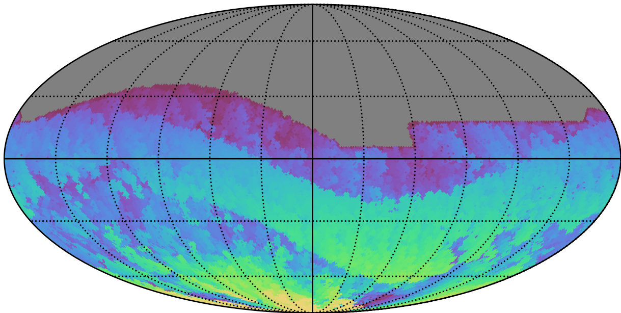
noroll_mjdp365_v3.4_10yrs All sky i band: Max HA
