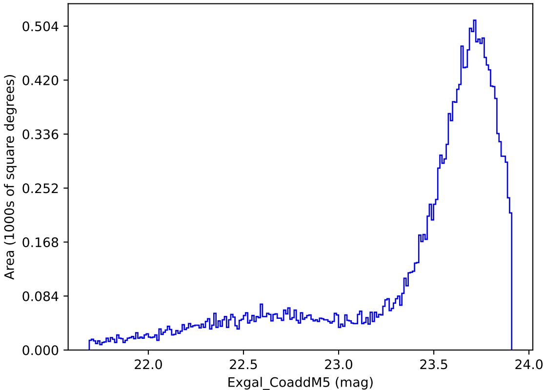
noroll_mjdp365_v3.4_10yrs Yr 1 y band: Exgal_CoaddM5
