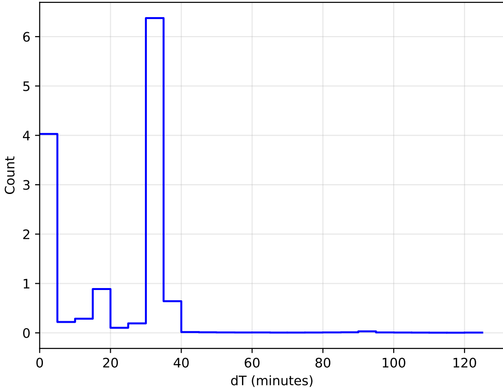
noroll_mjdp365_v3.4_10yrs All sky: DeltaT Histogram
