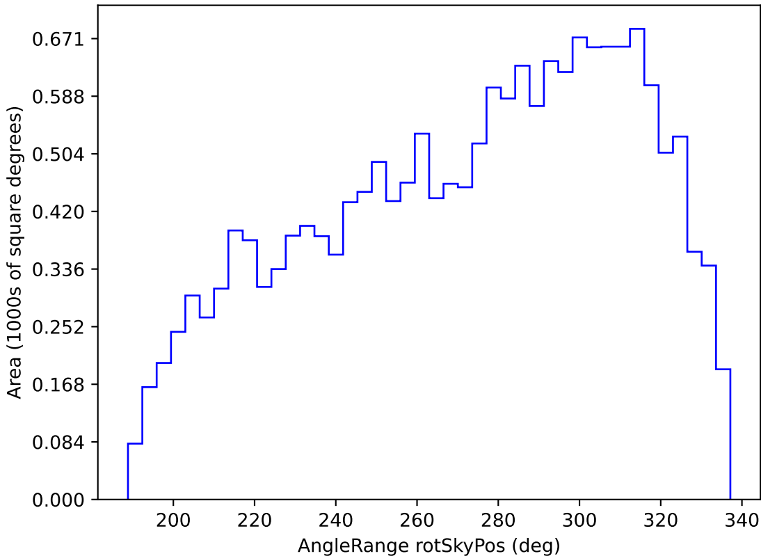
noroll_mjdp365_v3.4_10yrs WFD y band: AngleRange rotSkyPos
