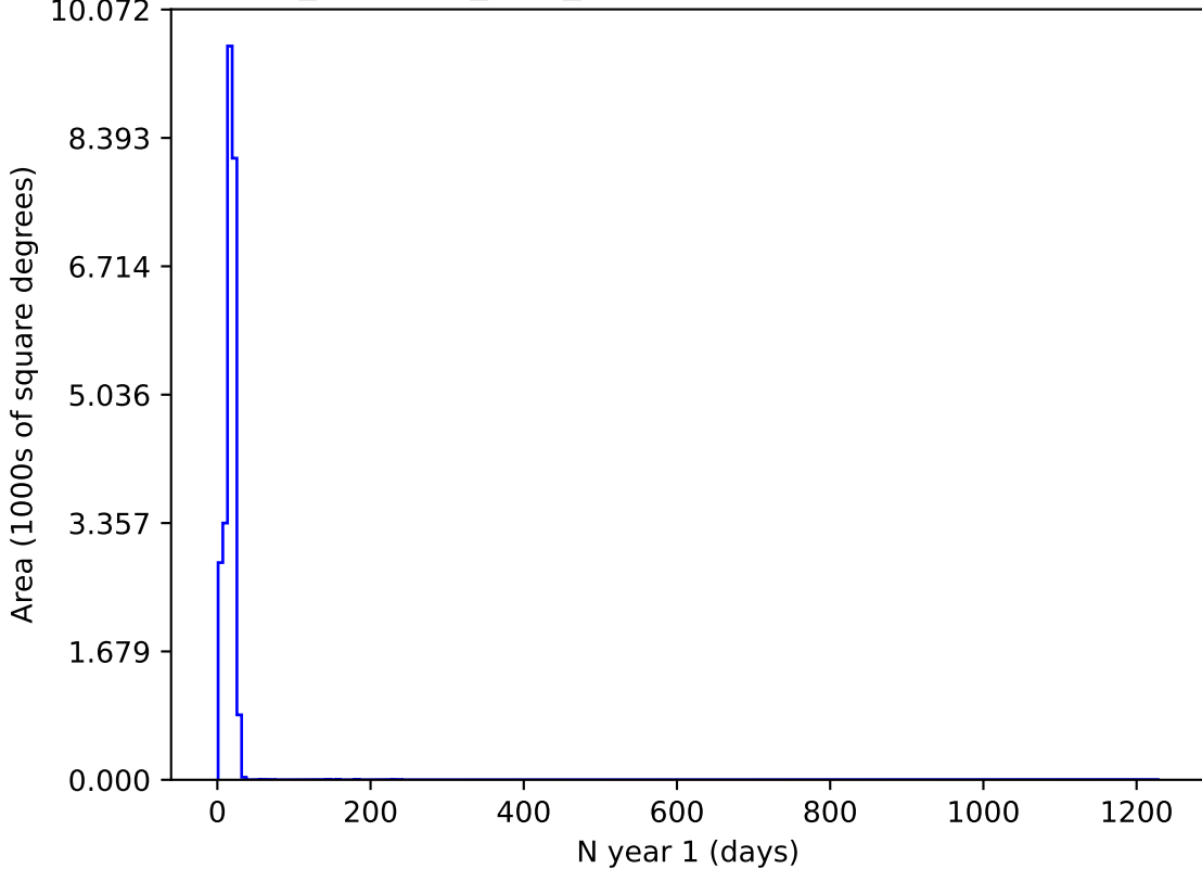
noroll_mjdp365_v3.4_10yrs y and night &lt; 365: N year 1
