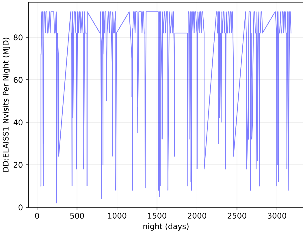
noroll_mjdp365_v3.4_10yrs all bands: DD:ELAISS1 Nvisits Per Night
