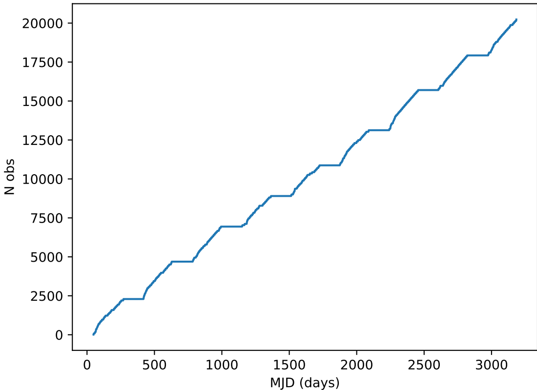
noroll_mjdp365_v3.4_10yrs all bands: DD:ELAISS1 Cumulative NVisits
