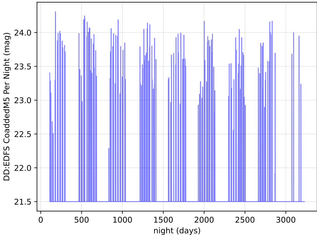
noroll_mjdp365_v3.4_10yrs y band: DD:EDFS CoaddedM5 Per Night
