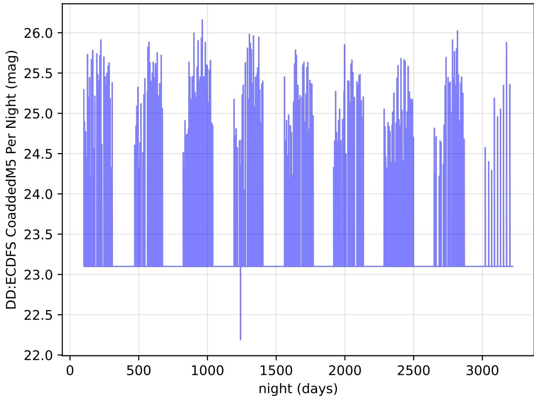
noroll_mjdp365_v3.4_10yrs i band: DD:ECDFS CoaddedM5 Per Night
