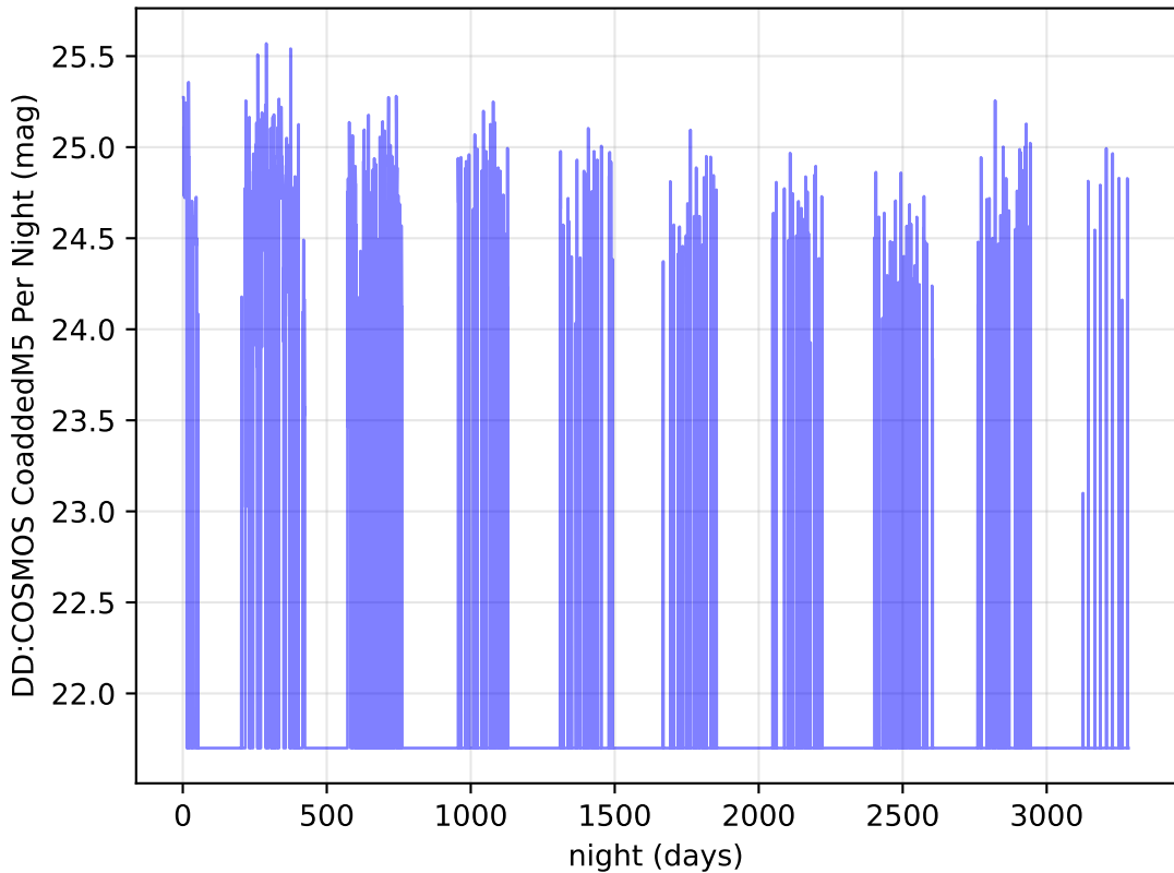
noroll_mjdp365_v3.4_10yrs z band: DD:COSMOS CoaddedM5 Per Night
