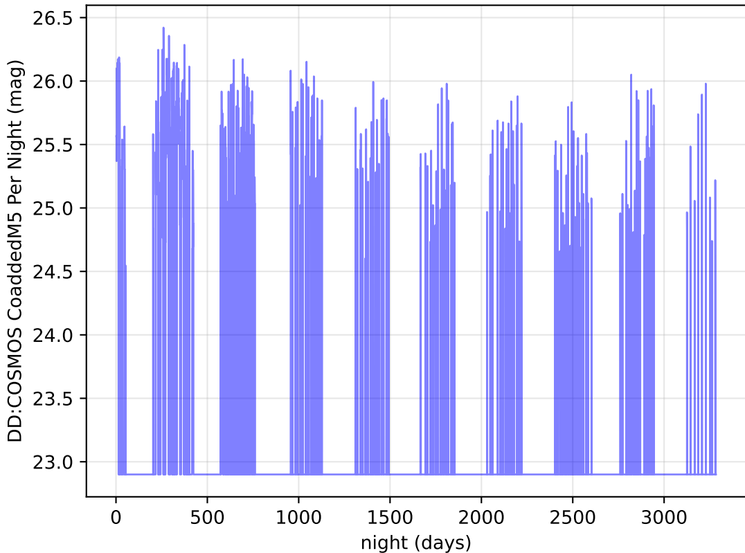
noroll_mjdp365_v3.4_10yrs r band: DD:COSMOS CoaddedM5 Per Night
