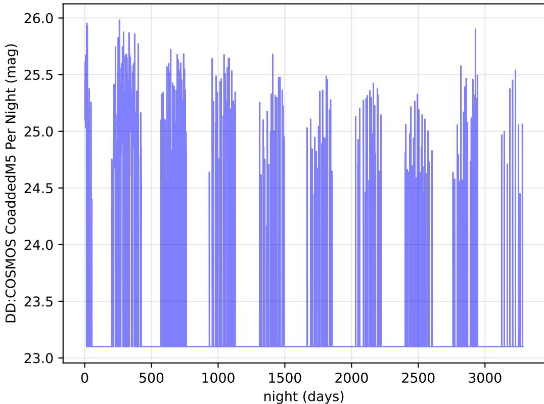
noroll_mjdp365_v3.4_10yrs i band: DD:COSMOS CoaddedM5 Per Night
