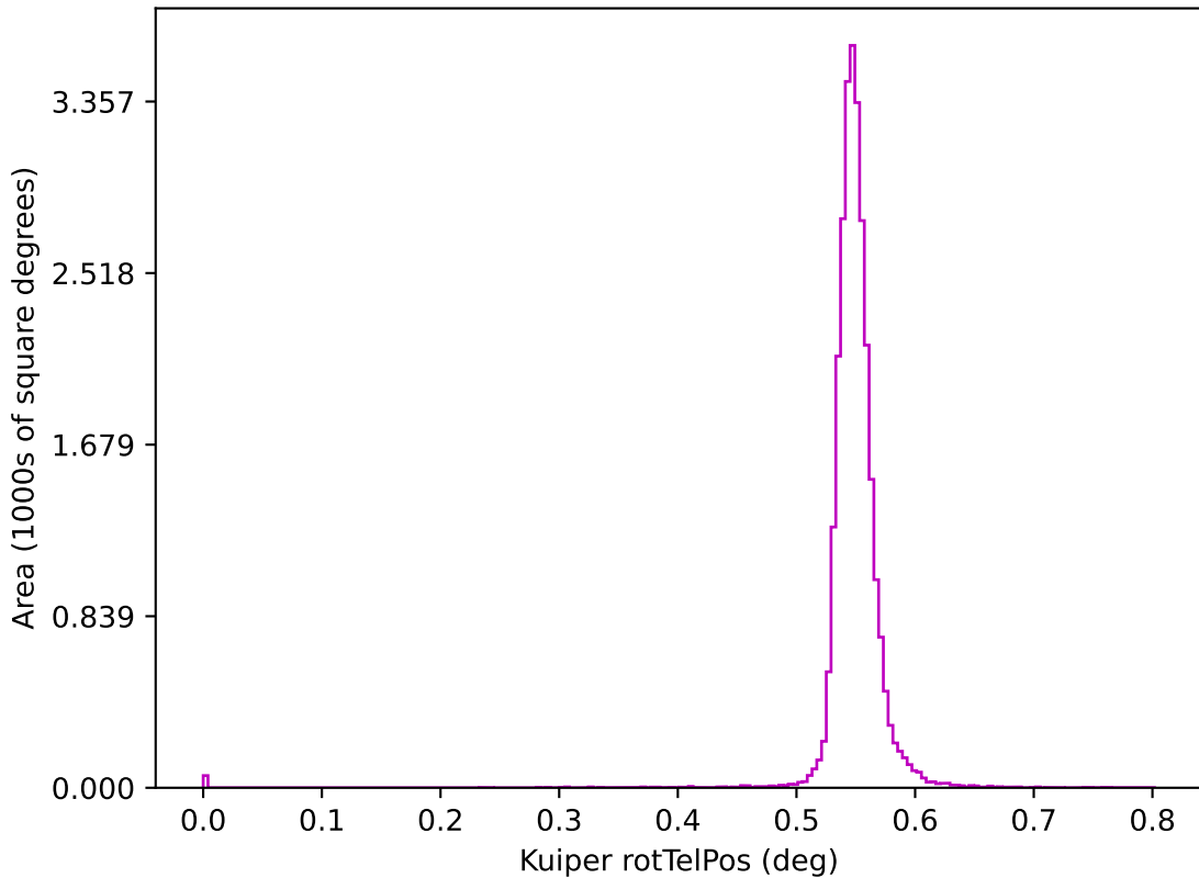
noroll_mjdp270_v3.4_10yrs z: Kuiper rotTelPos
