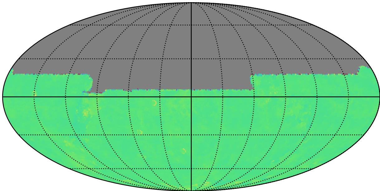
noroll_mjdp270_v3.4_10yrs y: Kuiper rotTelPos
