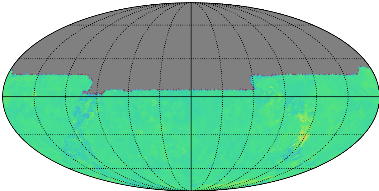
noroll_mjdp270_v3.4_10yrs u: Kuiper rotTelPos
