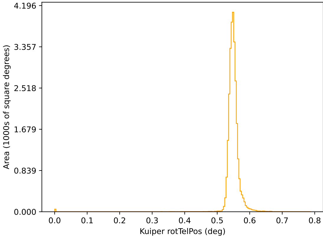
noroll_mjdp270_v3.4_10yrs r: Kuiper rotTelPos
