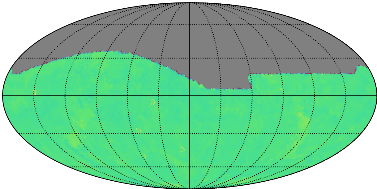
noroll_mjdp270_v3.4_10yrs g: Kuiper rotTelPos
