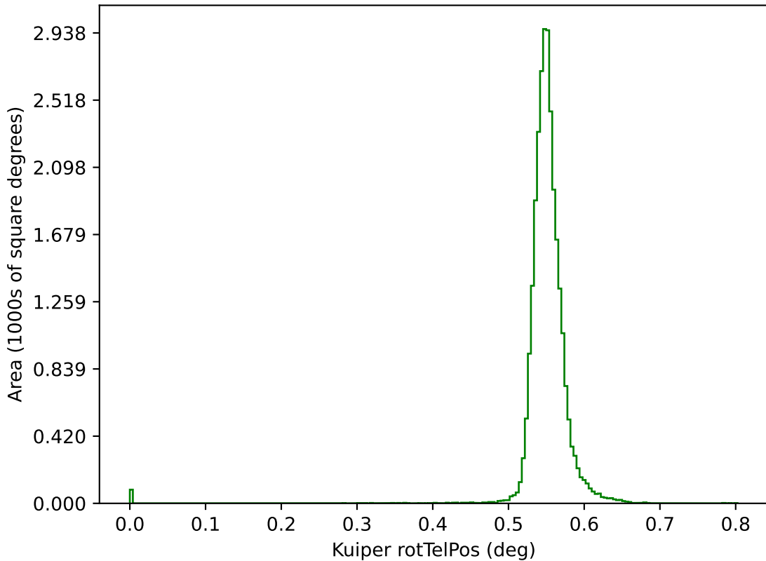
noroll_mjdp270_v3.4_10yrs g: Kuiper rotTelPos
