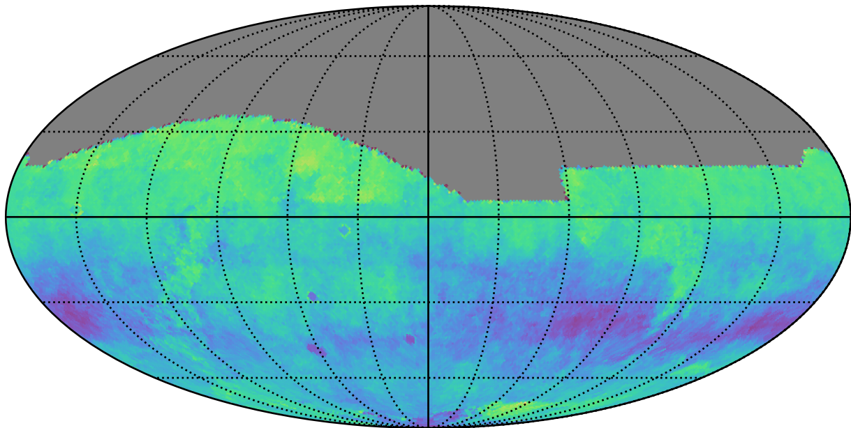
noroll_mjdp270_v3.4_10yrs z: Kuiper rotSkyPos
