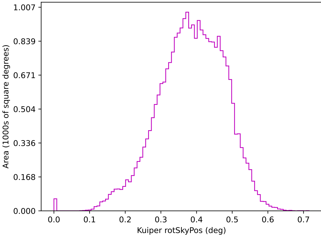
noroll_mjdp270_v3.4_10yrs z: Kuiper rotSkyPos
