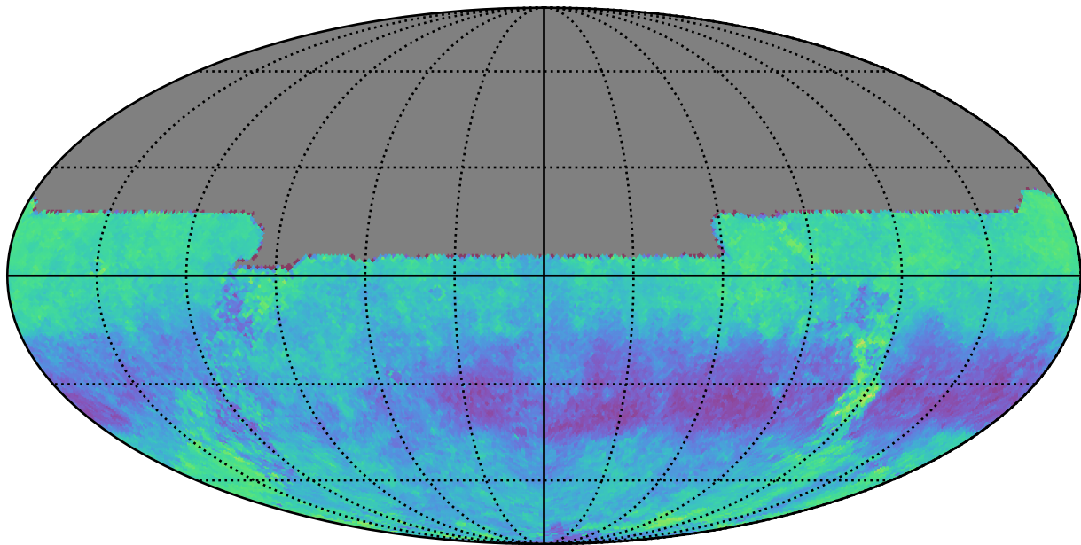
noroll_mjdp270_v3.4_10yrs u: Kuiper rotSkyPos
