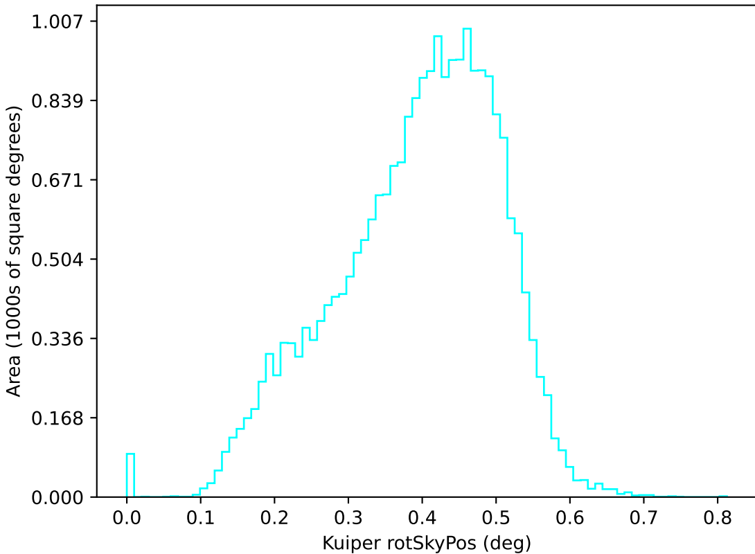
noroll_mjdp270_v3.4_10yrs u: Kuiper rotSkyPos
