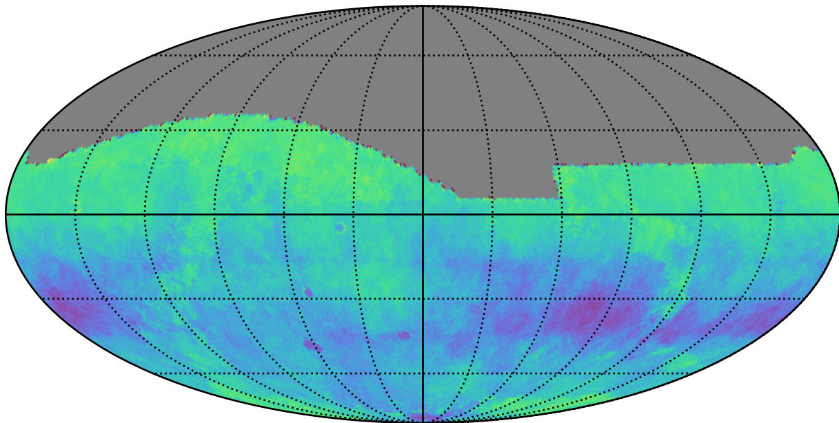
noroll_mjdp270_v3.4_10yrs i: Kuiper rotSkyPos
