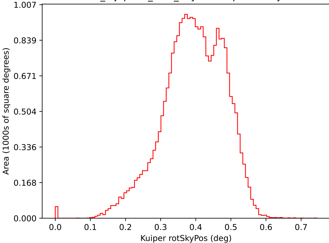
noroll_mjdp270_v3.4_10yrs i: Kuiper rotSkyPos
