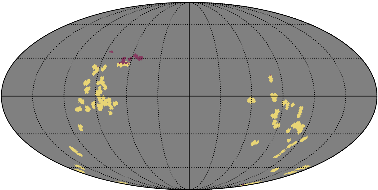
noroll_mjdp270_v3.4_10yrs : GalplaneFootprintMetric_zucker_sfr_map_Tau_46_5
