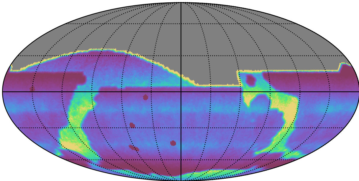
noroll_mjdp270_v3.4_10yrs : DCRprecision
