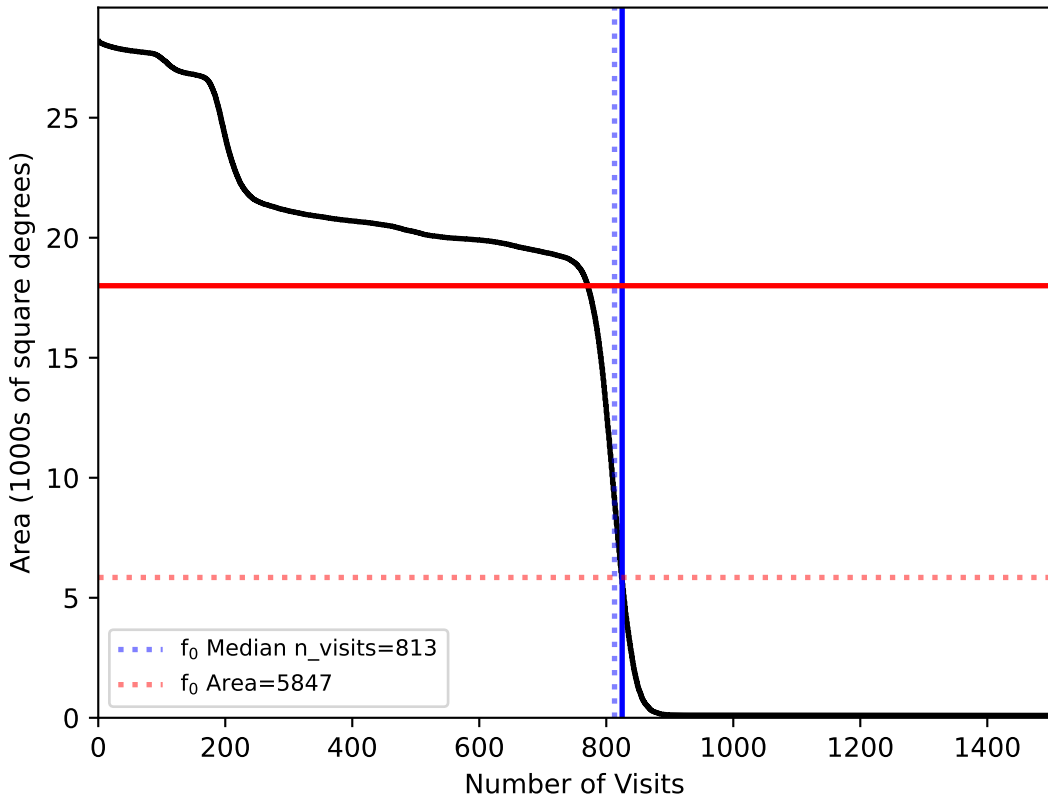
noroll_mjdp270_v3.4_10yrs All sky: f0
