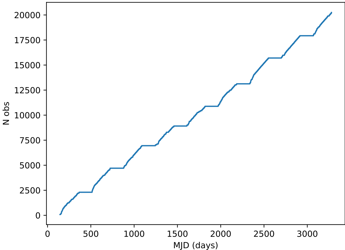
noroll_mjdp270_v3.4_10yrs note like DD:ELAISS1%: Cumulative
