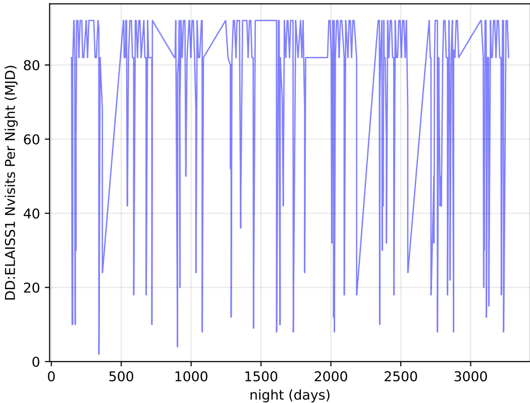
noroll_mjdp270_v3.4_10yrs all bands: DD:ELAISS1 Nvisits Per Night
