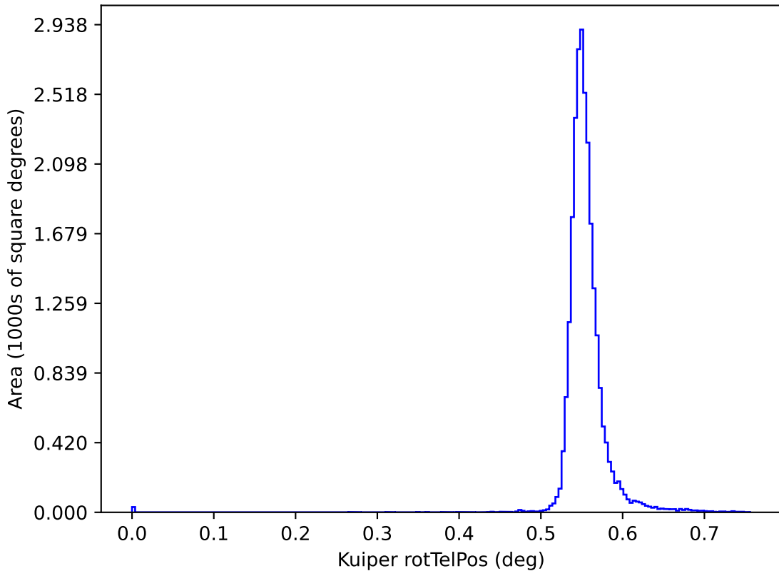
noroll_mjdp180_v3.4_10yrs y: Kuiper rotTelPos
