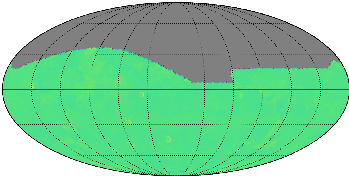
noroll_mjdp180_v3.4_10yrs i: Kuiper rotTelPos
