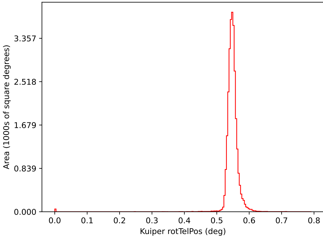
noroll_mjdp180_v3.4_10yrs i: Kuiper rotTelPos
