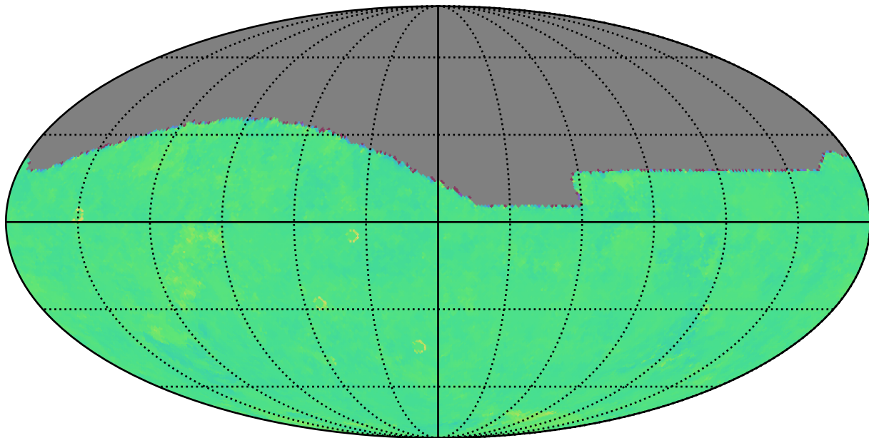
noroll_mjdp180_v3.4_10yrs g: Kuiper rotTelPos
