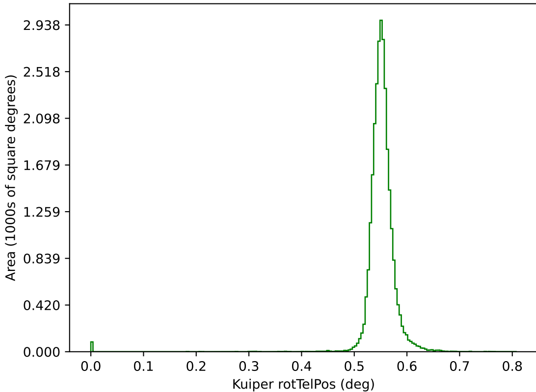
noroll_mjdp180_v3.4_10yrs g: Kuiper rotTelPos
