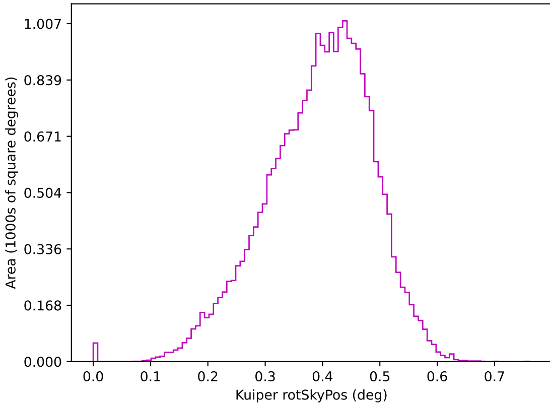
noroll_mjdp180_v3.4_10yrs z: Kuiper rotSkyPos
