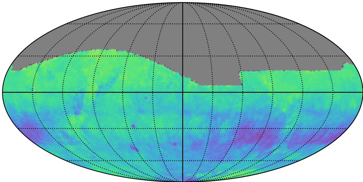
noroll_mjdp180_v3.4_10yrs i: Kuiper rotSkyPos
