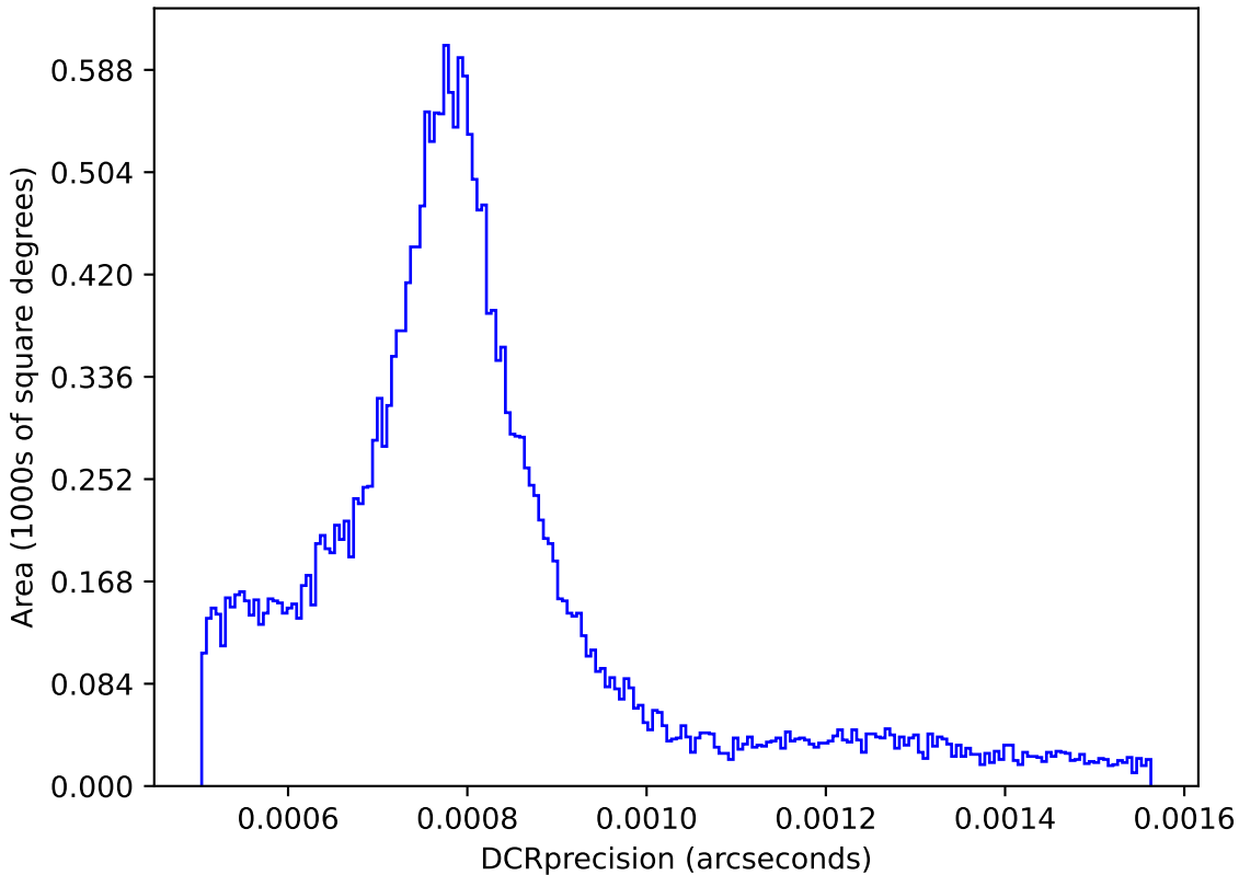
noroll_mjdp180_v3.4_10yrs : DCRprecision
