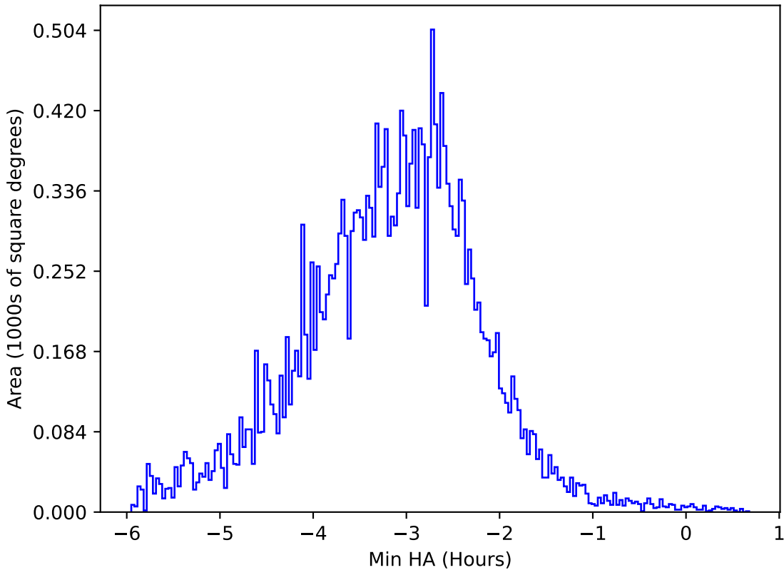
noroll_mjdp180_v3.4_10yrs All sky y band: Min HA
