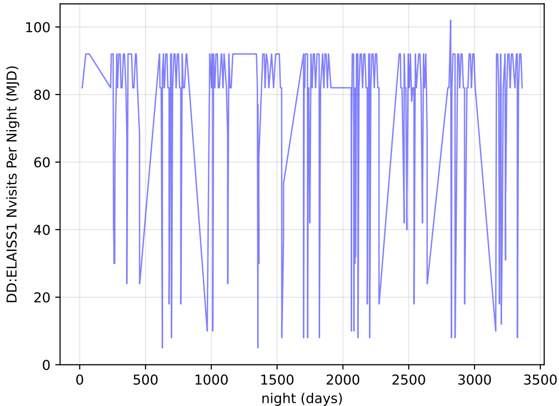
noroll_mjdp180_v3.4_10yrs all bands: DD:ELAISS1 Nvisits Per Night
