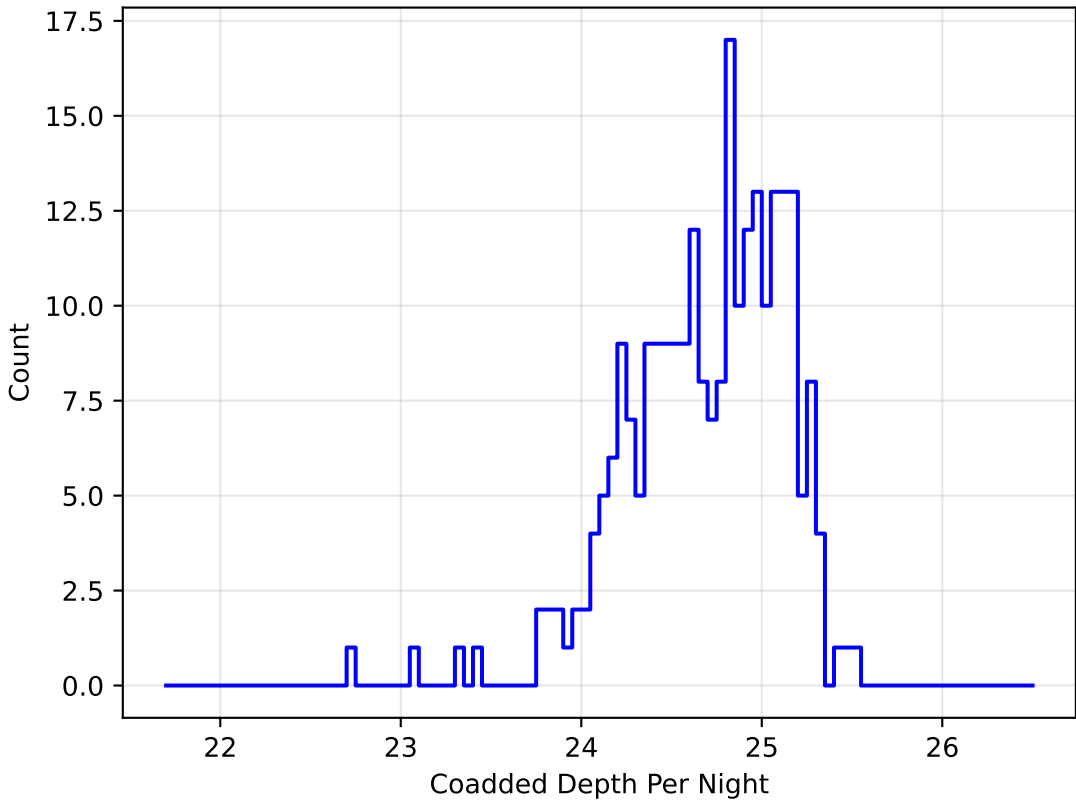
noroll_mjdp180_v3.4_10yrs z band: DD:EDFS CoaddM5PerNight
