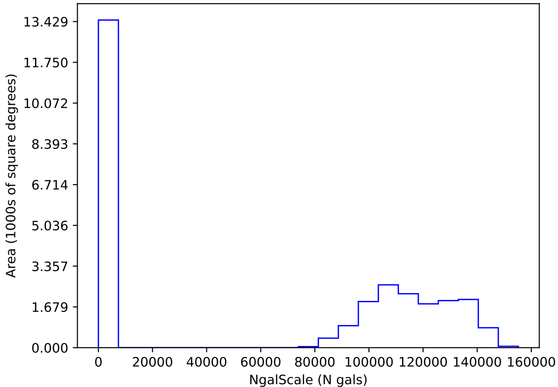
noroll_mjdp120_v3.4_10yrs i: NgalScale
