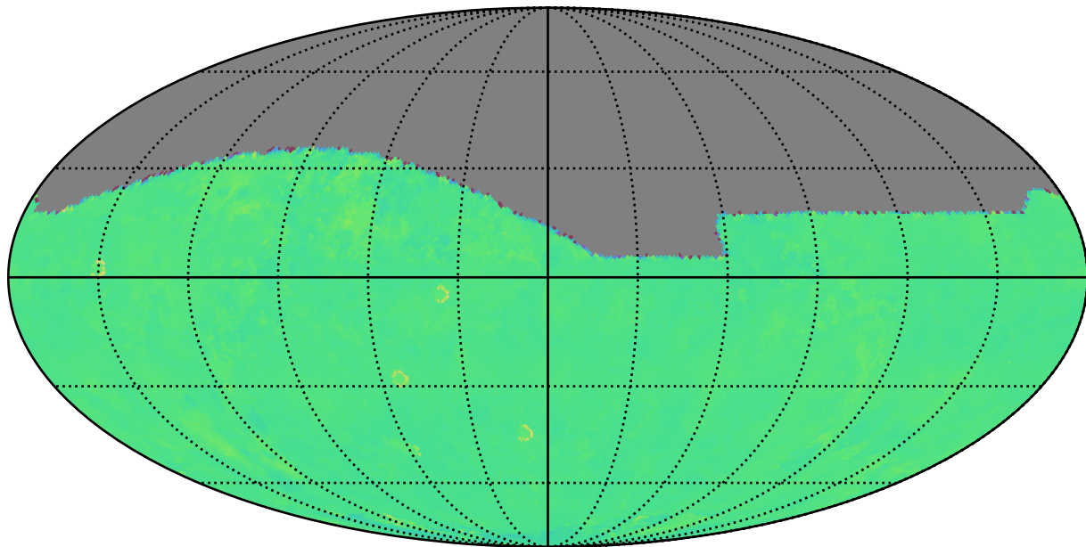
noroll_mjdp120_v3.4_10yrs z: Kuiper rotTelPos
