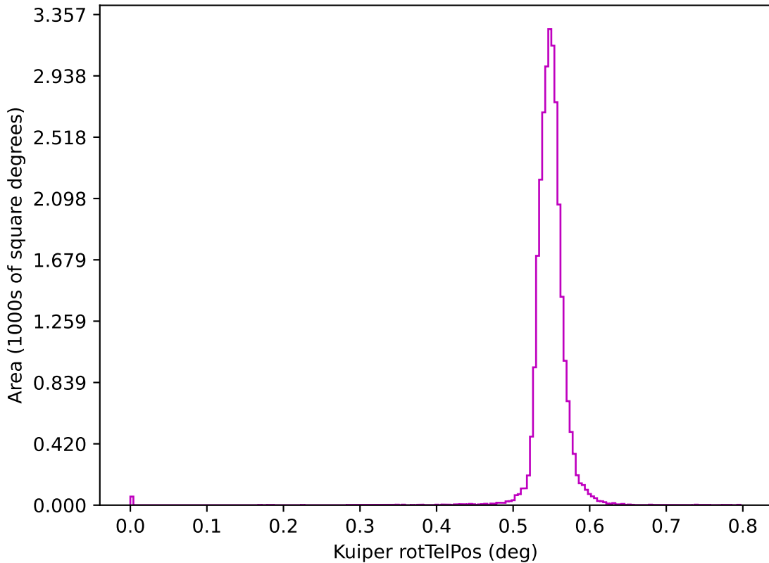
noroll_mjdp120_v3.4_10yrs z: Kuiper rotTelPos
