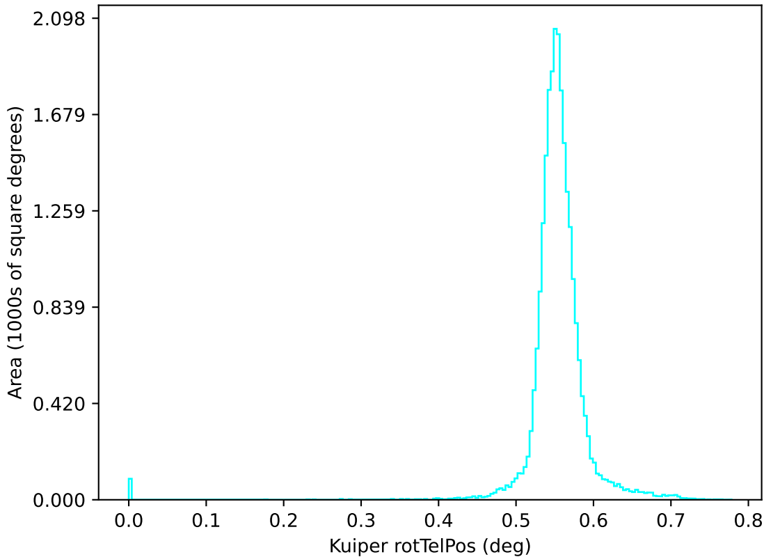
noroll_mjdp120_v3.4_10yrs u: Kuiper rotTelPos
